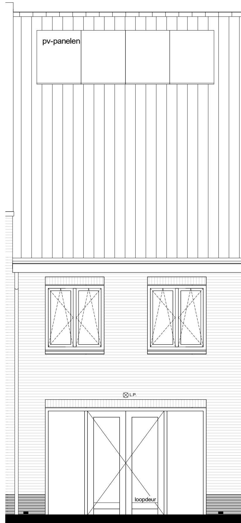
achtergevel
