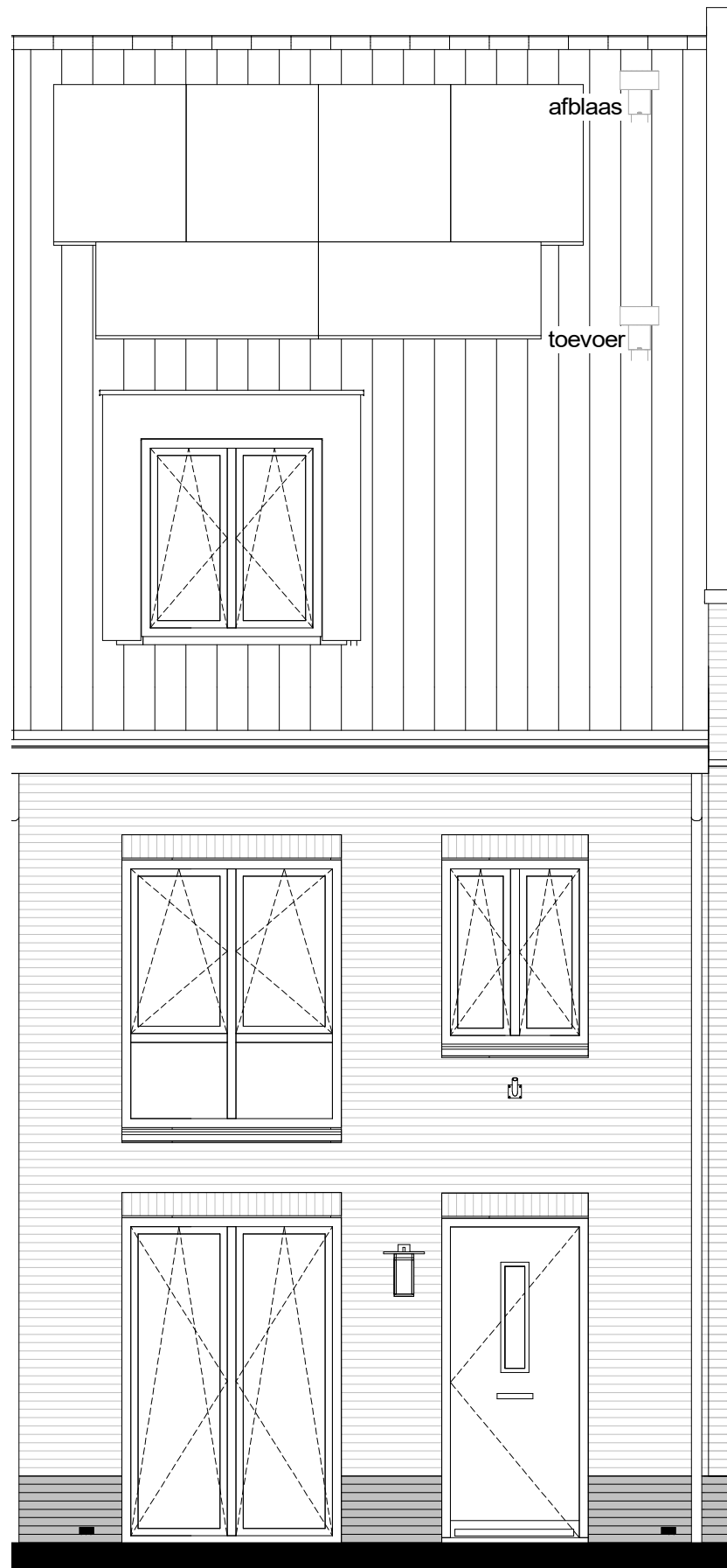
voorgevel
