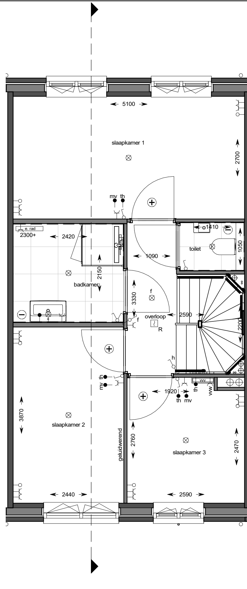
eerste verdieping
